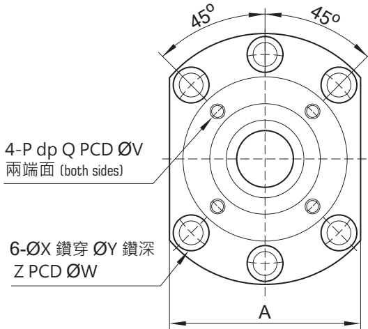
軸徑 Ød = 30 Shaft diameter
