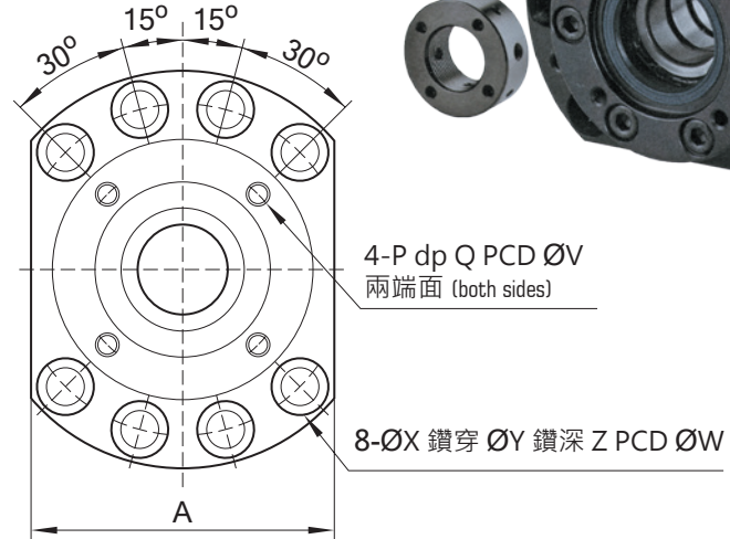
軸徑 Ød = 30 Shaft diameter
